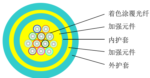
数据中心光缆 II 型
